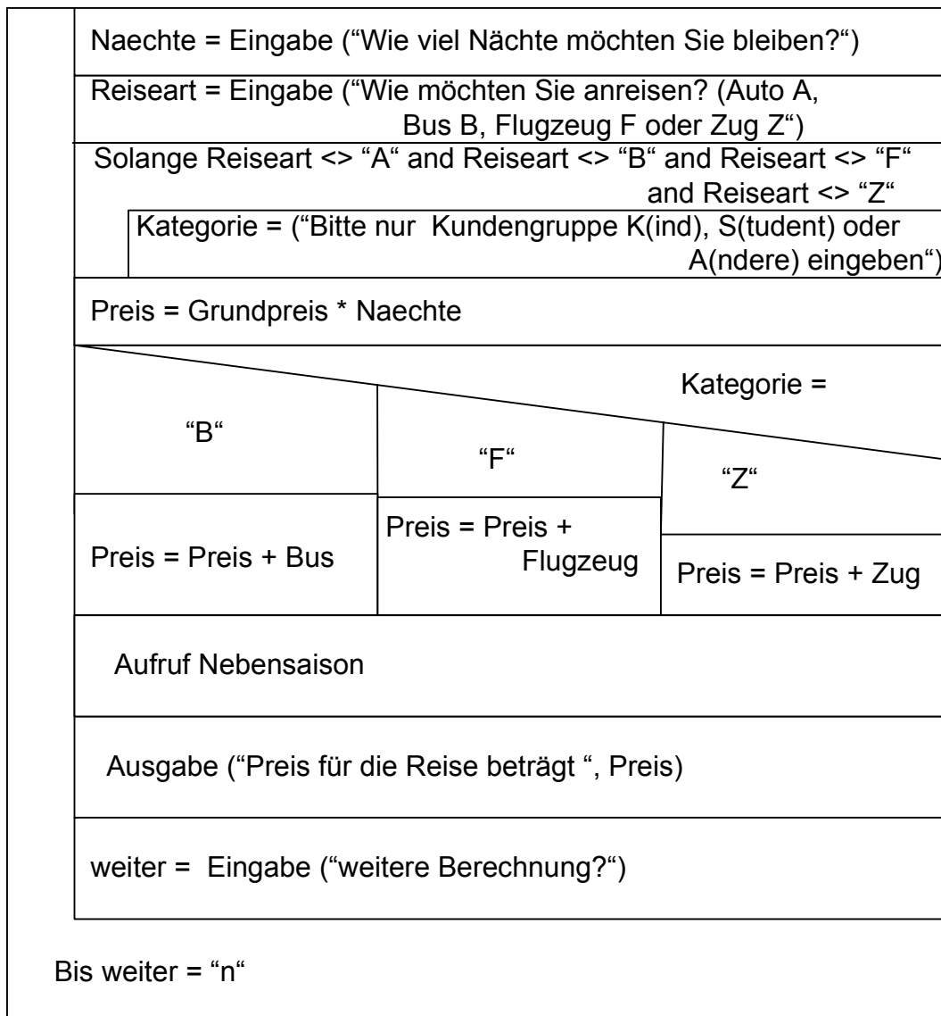
Struktogramm zum Hauptprogramm der Aufgabe 4.1 "Parisreise"
