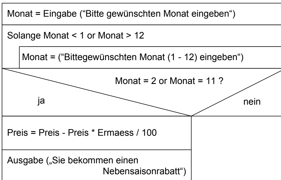
Struktogramm zum Unterprogramm der Aufgabe 4.1 "Nebensaison"
